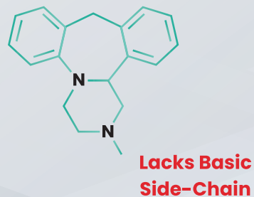
Mianserin
